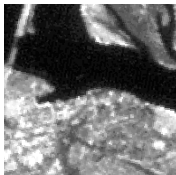
Рис. 5. Собственная яркость объектов спектрального канала 0.78 мкм – 0.86 мкм.
