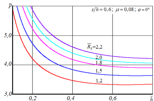
Рис. 6. Залежність тиску послідовного комбінованого видавлювання від відносної висоти \bar{h} і радіусу порожнини \bar{R}_3 при s/h = 0,6
